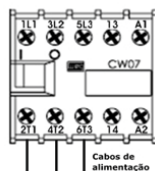
Entre com os cabos na parte inferior
