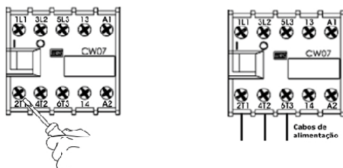
Solte os 03 parafusos do contator
