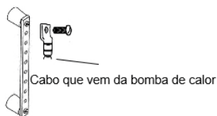
conector no barramento do quadro de distribuição
