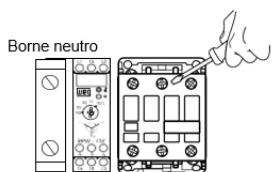
Solte os 03 parafusos do contator E os parafusos do borne NEUTRO
