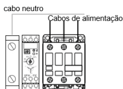
entre com os cabos na parte superior e alimentar o Borne NEUTRO
